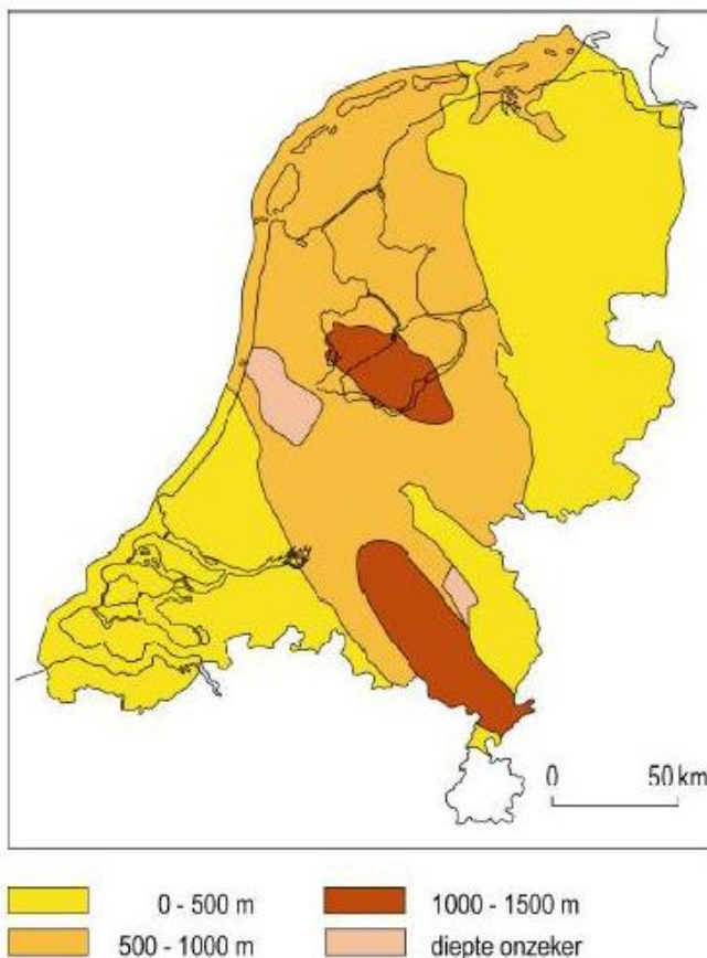
Figuur 5.1 Kleilagen Nederland
