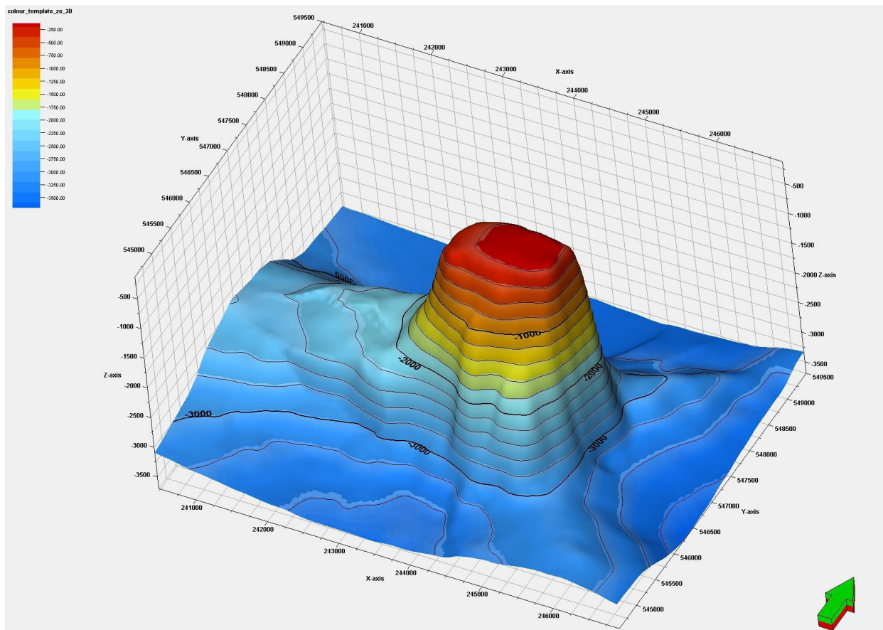
Figuur 4.15 Ligging zoutkoepel Schoonloo
