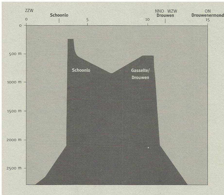
Figuur 4.9 Ligging zoutkoepel Gasselte
