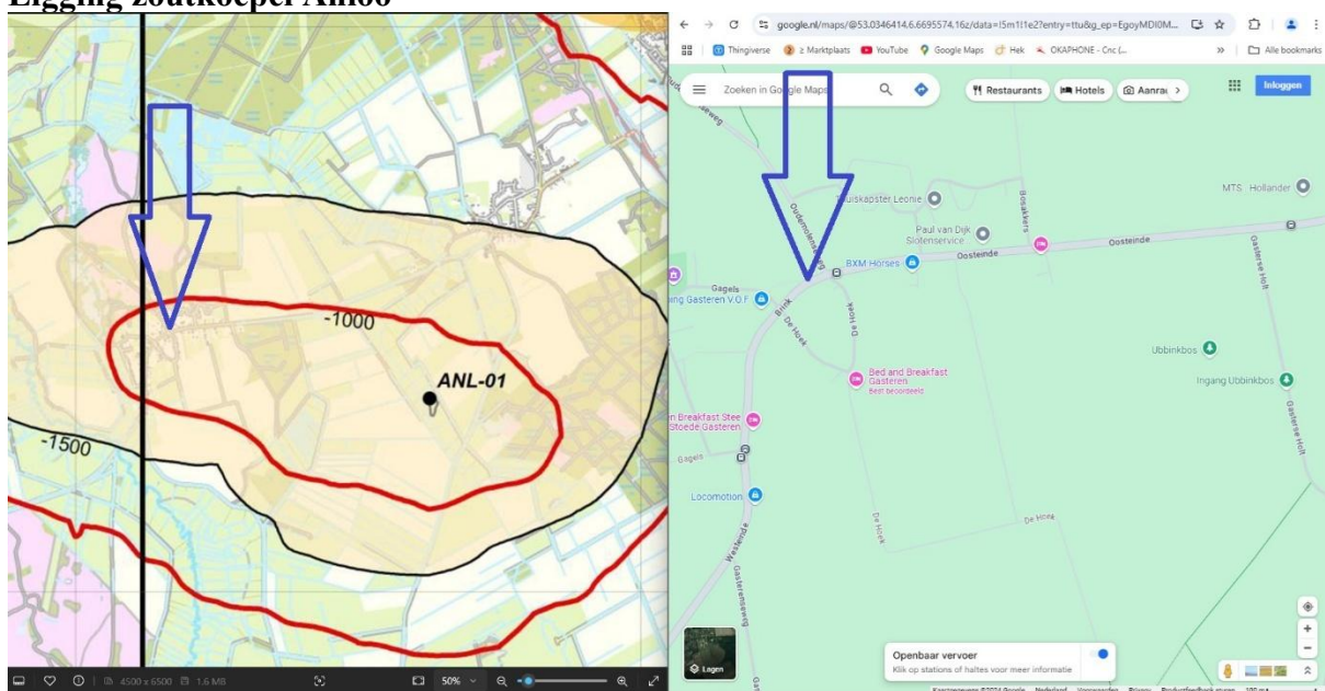
Figuur 4.6 Zoutkoepel Bourtange
