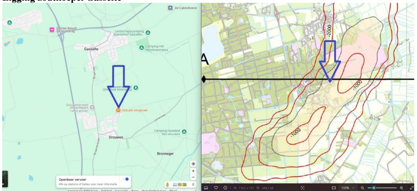
Figuur 4.9 Ligging zoutkoepel Gasselte
