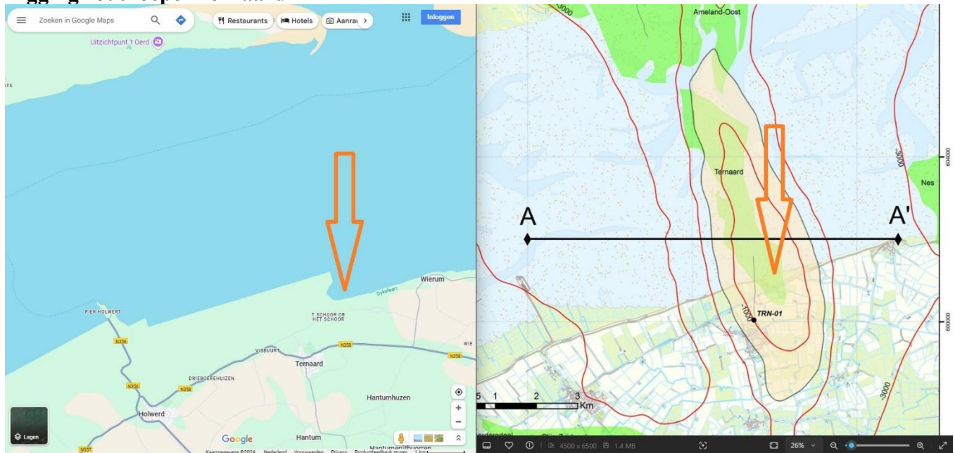
Figuur 4.18 Zoutkoepel Hooghalen
